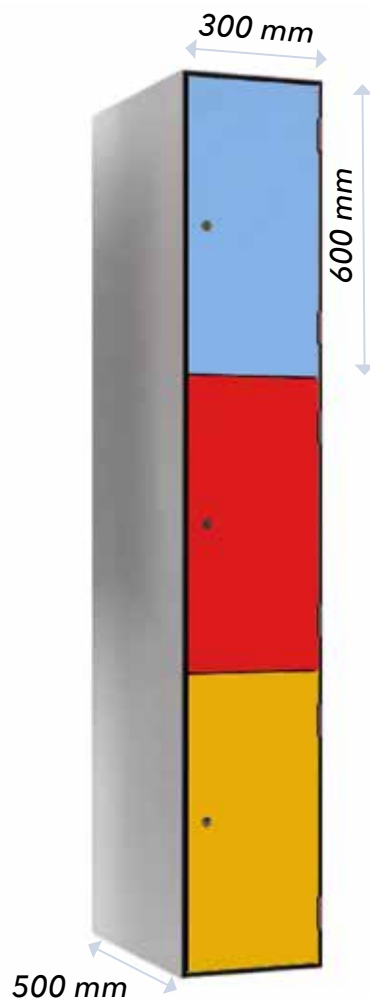
Colonne 3 casiers
